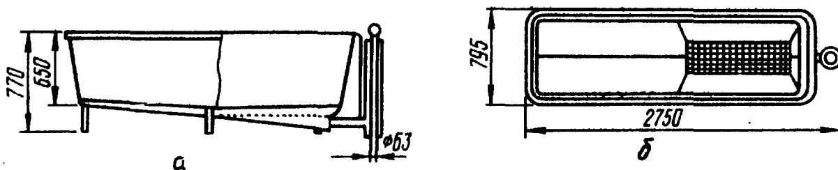
Рис. 11. Стеклопластиковый прямоточный бассейн для молоди:
