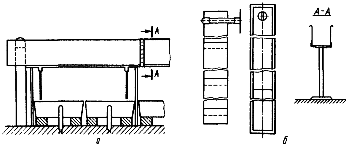
Рис. 14. Водораспределительные устройства :
